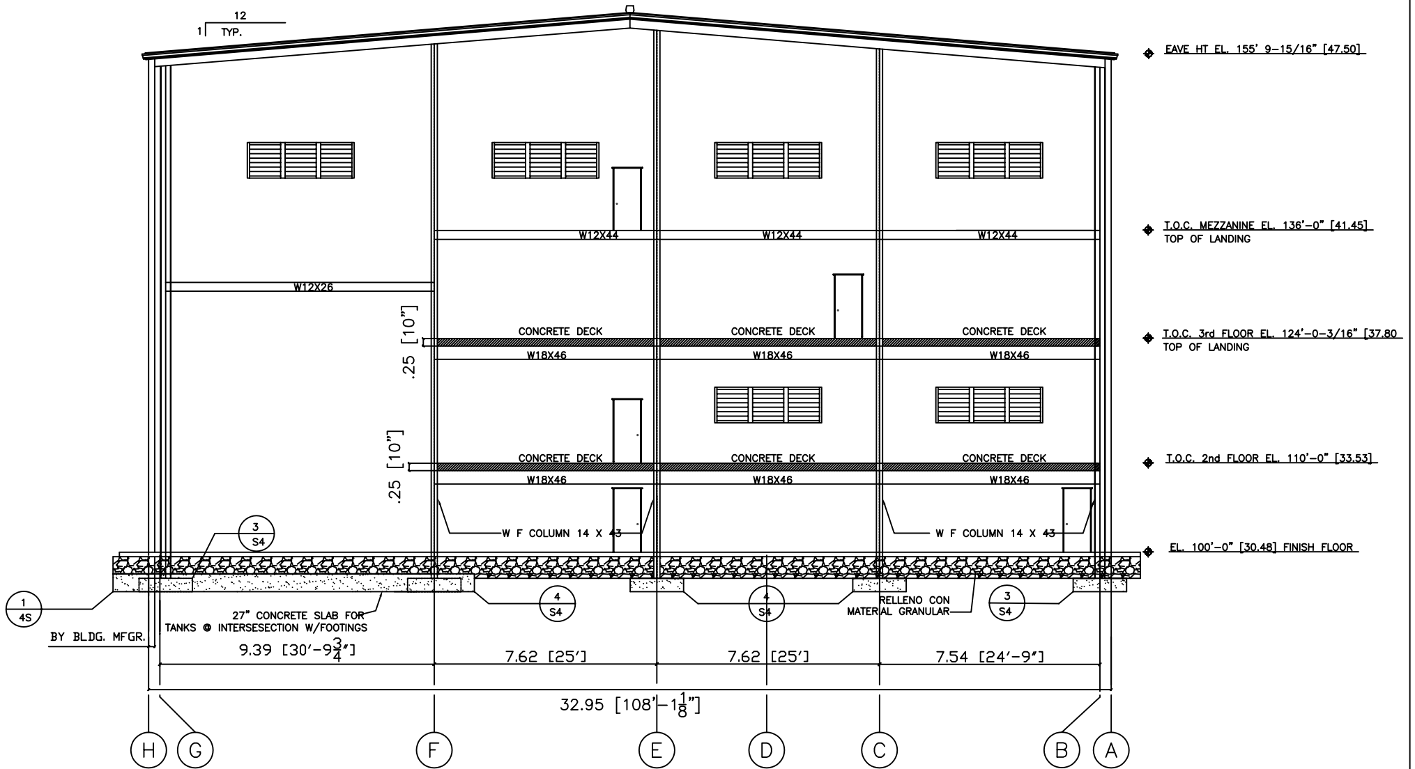
Elevacion Posterior
